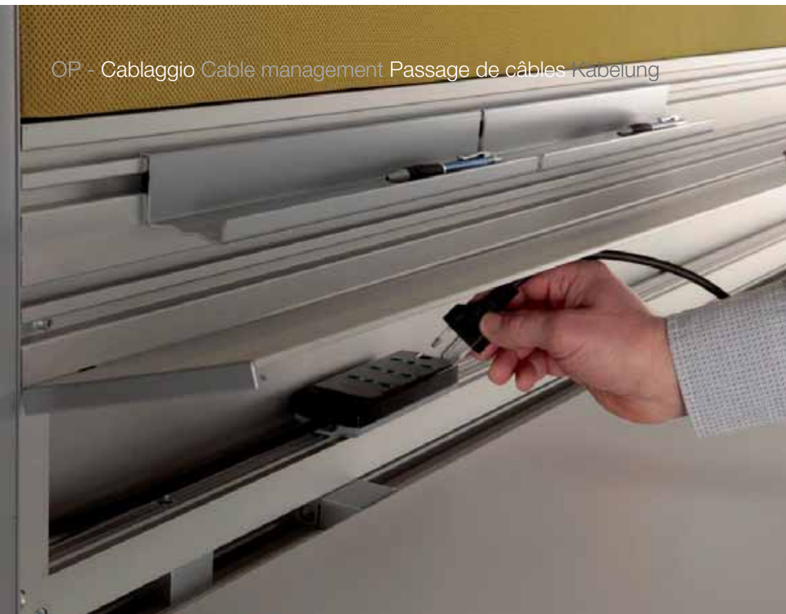
Schermo con spina tecnica cablata e canalizzazione verticale Screen with wired technical duct and vertical cable management
